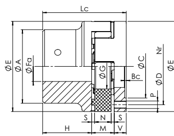
albero - flangia
