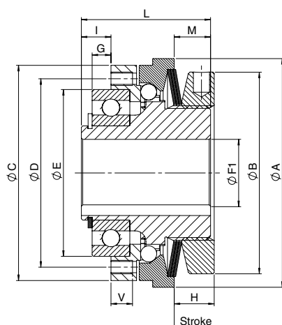
Versione con foro e cava
