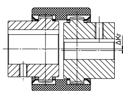
disallineamento radiale
