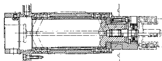
Anello elastico
